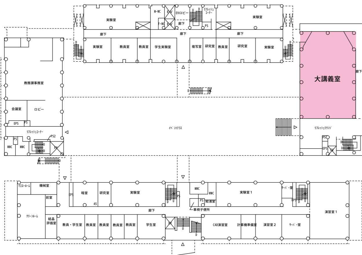
2階
